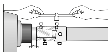
Соединение кабелей в диапазоне одной ступени стандартных сечений кабелей при использовании специального соединителя
